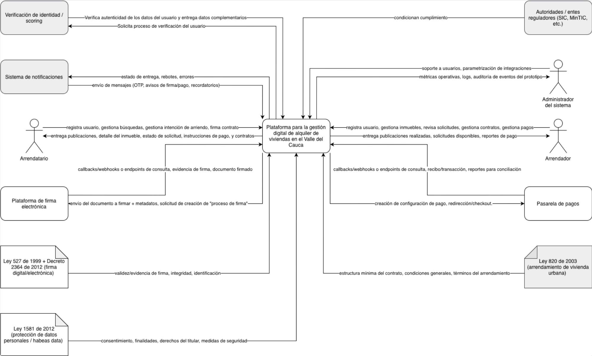
Desde el punto de vista arquitectónico se plantea este primer acercamiento a la vista de contexto del modelo C4:
